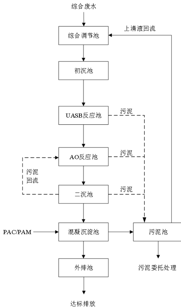
图 4.1-1 环评阶段综合废水处理工艺流程图
