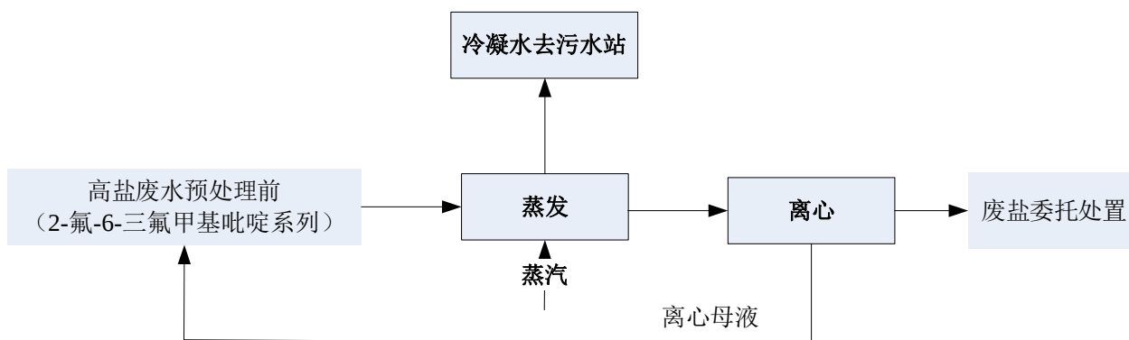
图 4.1-2 2-氟-6-三氟甲基吡啶系列高盐废水预处理工艺流程图
