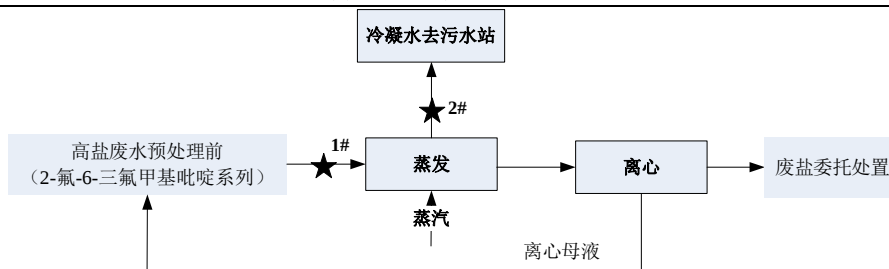
图 7.1-1 2-氟-6-三氟甲基吡啶系列高盐废水预处理工艺流程图
