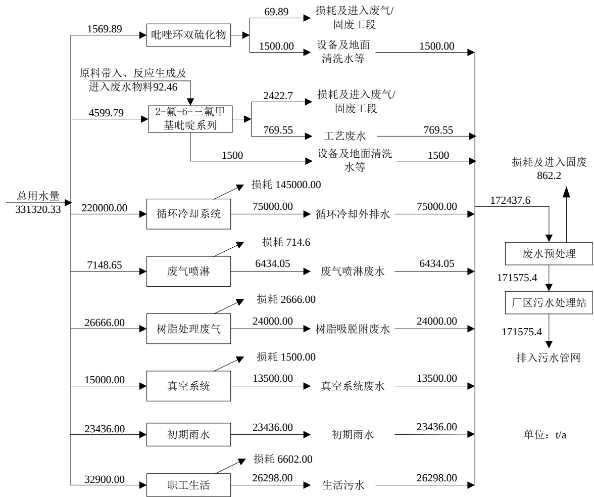
图 3.5-1 项目水平衡图
