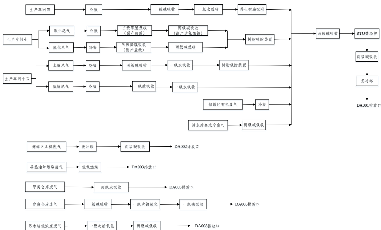
图 4.1-4 项目本期建设内容废气处理工艺流程
