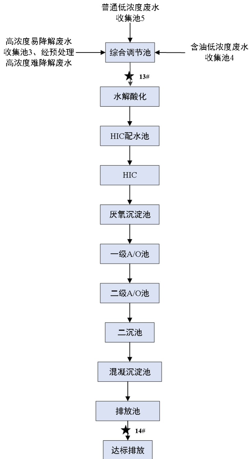
图 7.1-2 8#普通低浓度废水处理工艺流程图
