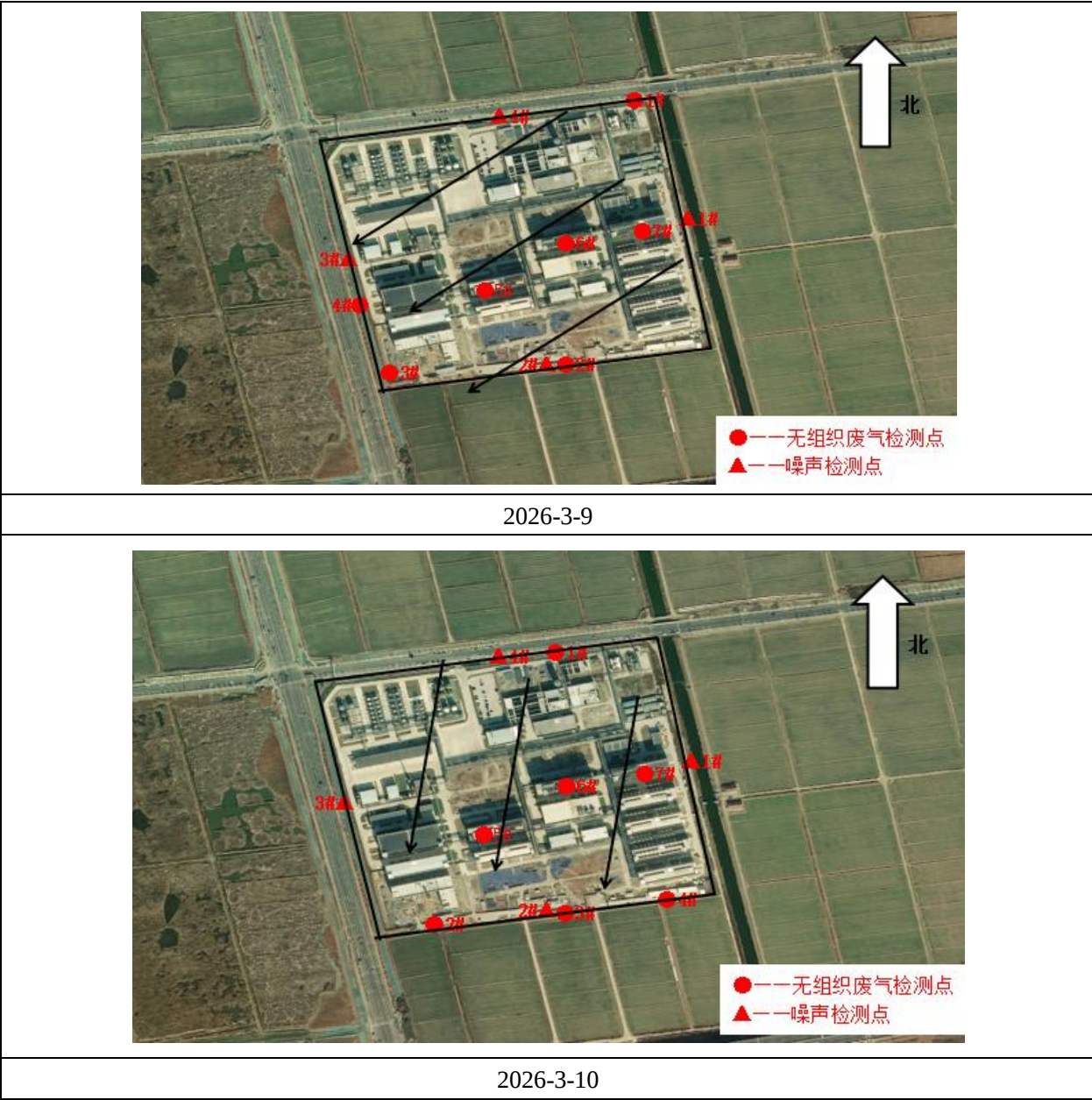
图 7.1-4 无组织废气及噪声监测布点图
