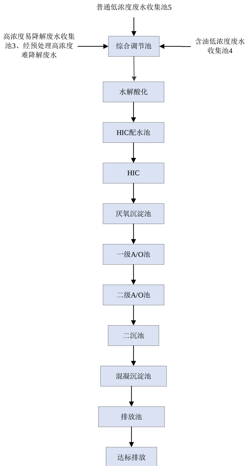
图 4.1-3 综合废水处理处理工艺流程
